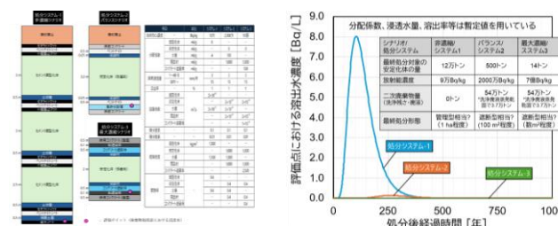
三つの処分システム(案)およびパラメータ(左)と評価点における浸出水の経時変化(計算例)(右)
