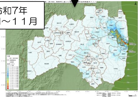
空間線量率マップ
