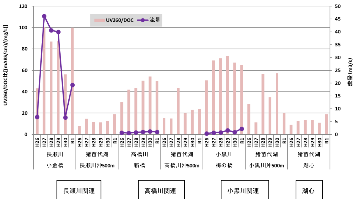
図 6 平成 26 年度から令和元年度の UV260/DOC 比及び流量
