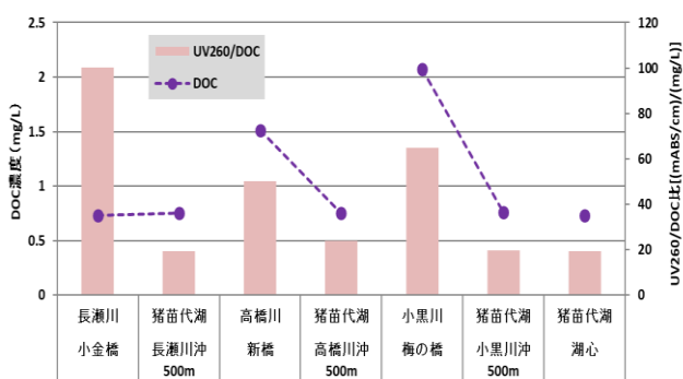
図 5 UV260/DOC 比及び DOC 濃度
