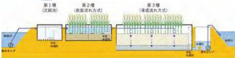
図4 人工湿地の構造
